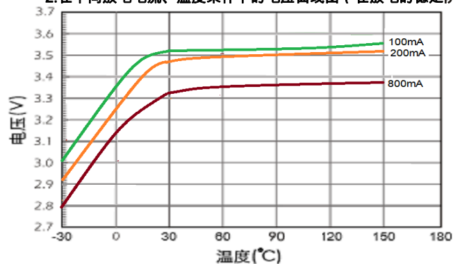
2. 在不同放电电流、温度条件下的电压曲线图 (在放电的稳定阶段)
