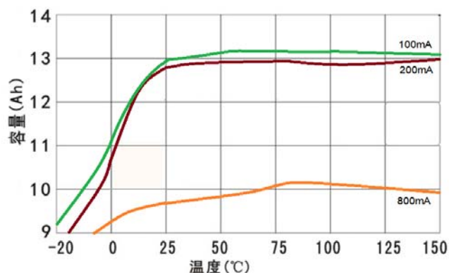
3. 在不同温度和电流条件下的容量曲线图 (截止电压为 2.0V)
