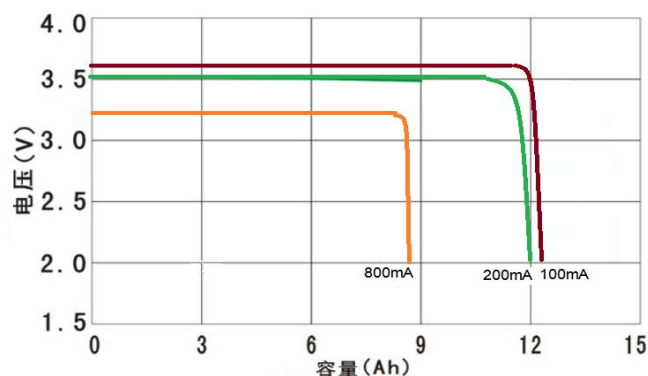
1. 在+135℃下典型放电曲线 (中间值)
